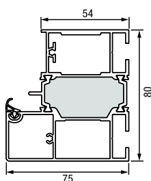
Huisserie A4
